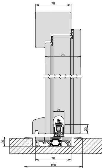
Set Comfort-Plan® 78 1-křídle
