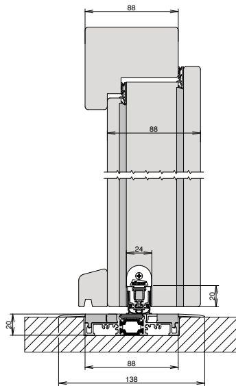
Set Comfort-Plan® 88 1-křídle
