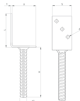
PATKA SLOUPKU OTEVŘENÁ LBOT
