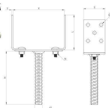
PATKA SLOUPKU STAVITELNÁ LBREG
